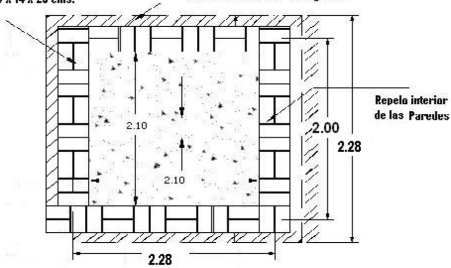
PLANTA ESTRUCTURAL
