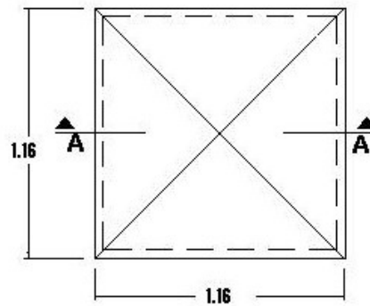
DETALLE DE TAPADERA METALECA, PARA RECAMARA DE LOS DESECHOS INFECCIOSOS
