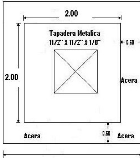
PLANIMETRIA DE CELDA PARA DESECHOS
