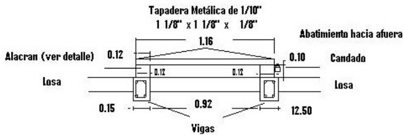
DETALLE DE TAPADERA METALECA, PARA RECAMARA DE LOS DESECHOS INFECCIOSOS
