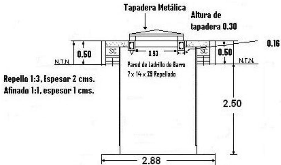
CELDA DE DESECHOS PATOLOGICOS SECCIÓN B - B
