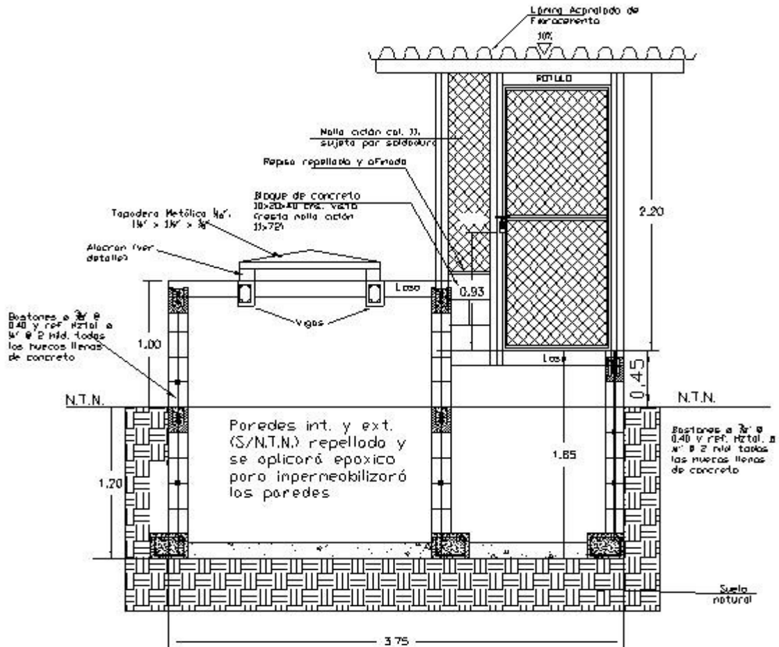
CELDA DE DESECHOS BIOPERCICIOSOS SECCIÓN A-A
